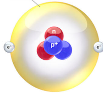
ذرة الهيليوم
