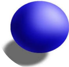
نموذج دالتون
