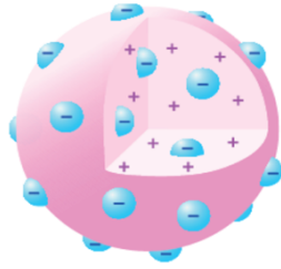
نموذج تومسون
