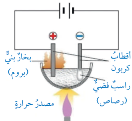
التحليل الكهربائي لمصهور بروميد الرصاص .
